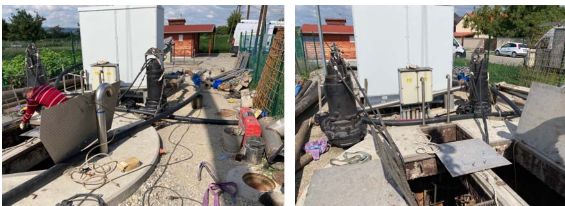
Kópháza A9 átemelő szivattyú rögzítés átépítés
