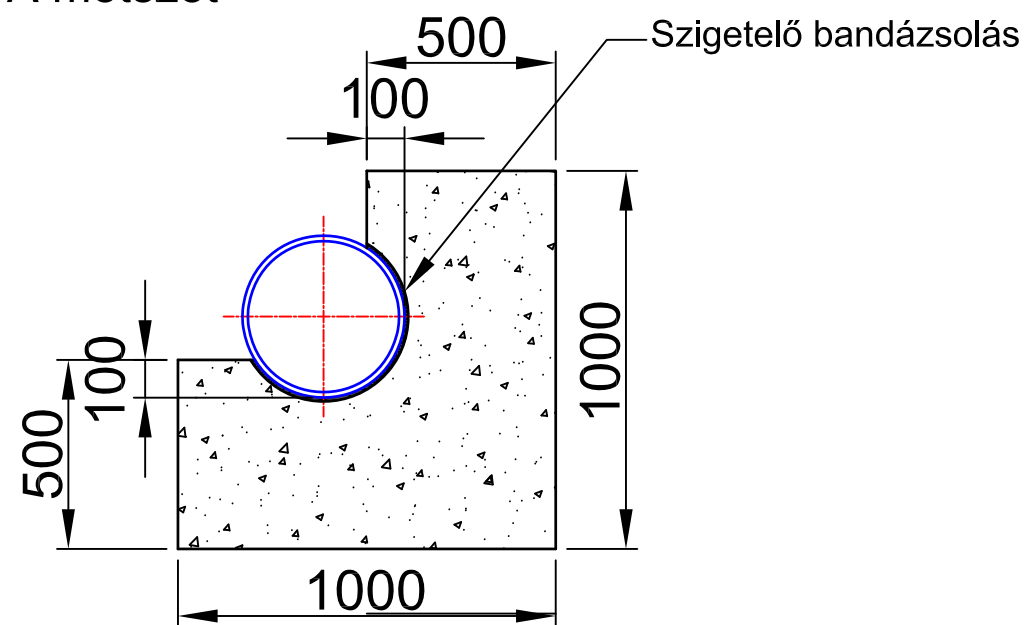
A - A metszet
