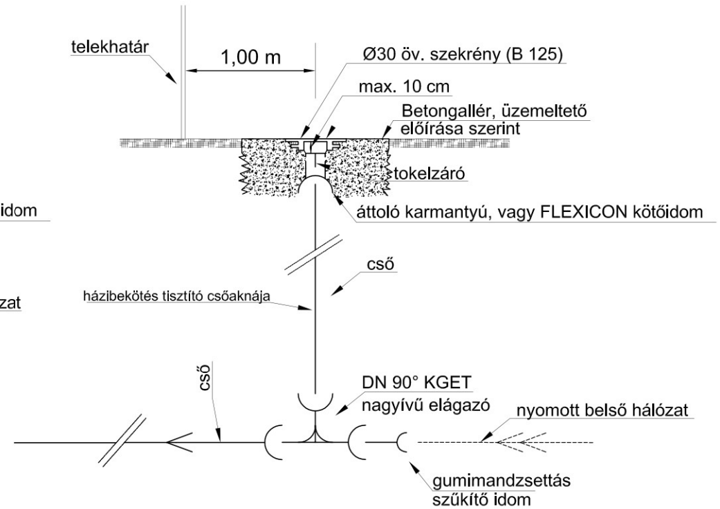
szennyvízbekötés és tisztítóidom részletrajza Egyenes átfolyású tisztítóval
