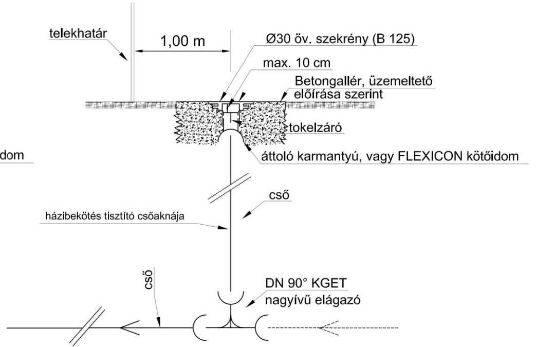
szennyvízbekötés és tisztítódóm részletrajza Egyenes átfolyású tisztítóval
